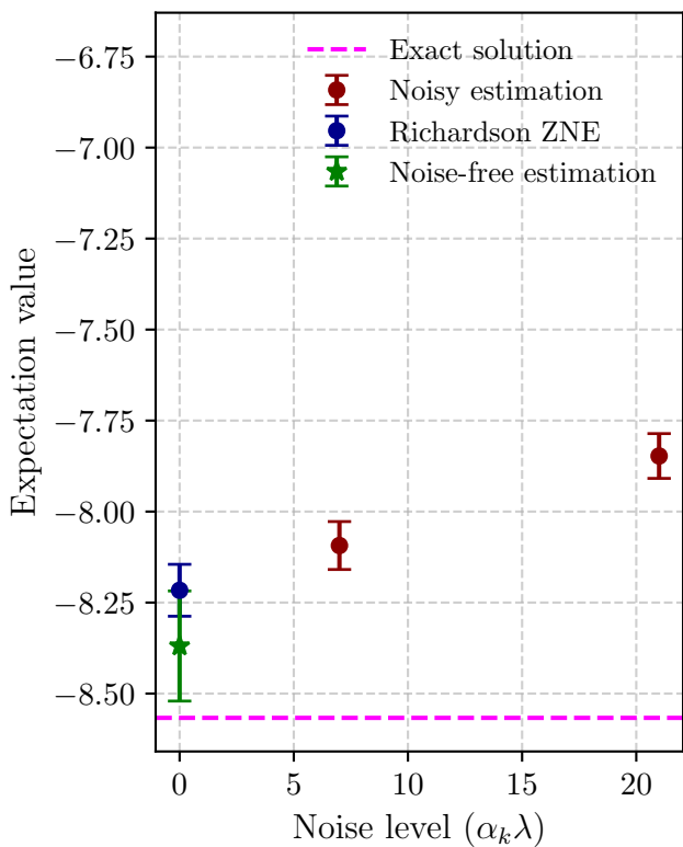
XY ansatz ric-5
